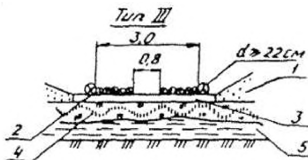
Графическая схема 2. Усиление ледовых переправ деревянным настилом:
